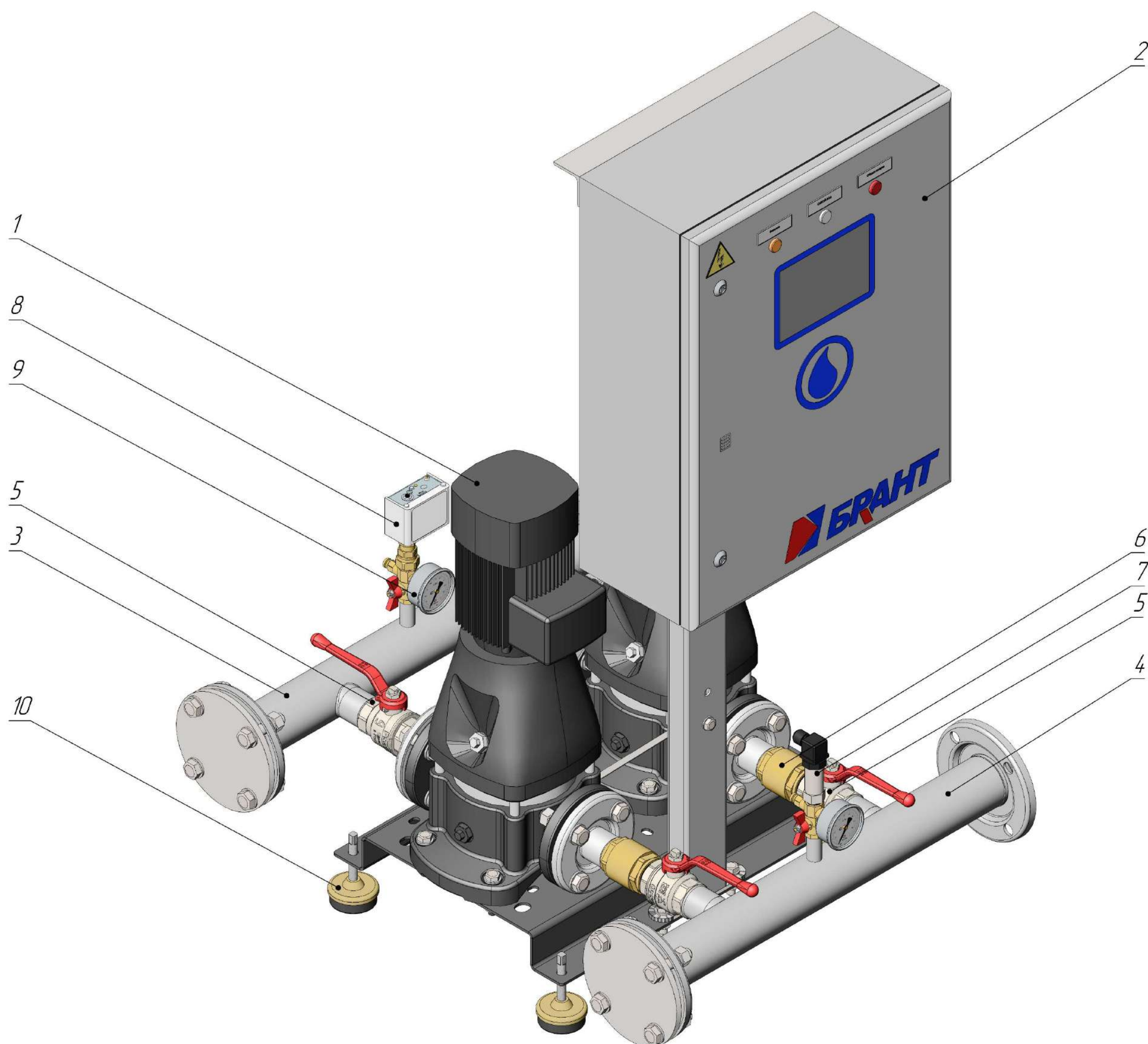
Рисунок – 14. Основное оборудование насосной установки серии Ч:
